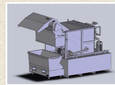
真空带式过滤机 (机床行业)
